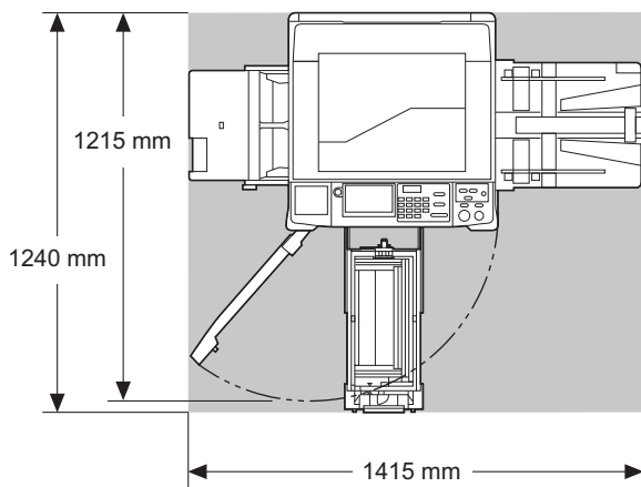
頂視圖
